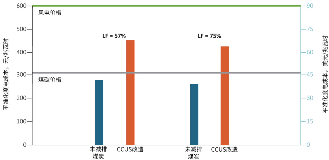
图 20 不同负载系数下未减排燃煤电厂和 CCUS 改造项目的 LCOE，给出平均煤炭价格（国家能源集团 2018 年的单位平均值）以及风电价格（华能风力电厂 2017 年的平均值）以进行比较
