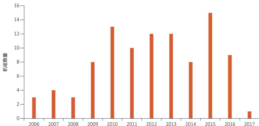
图 12 按照投入运转年份给出的中国 100 万千瓦机组 (Platts, 2018)
